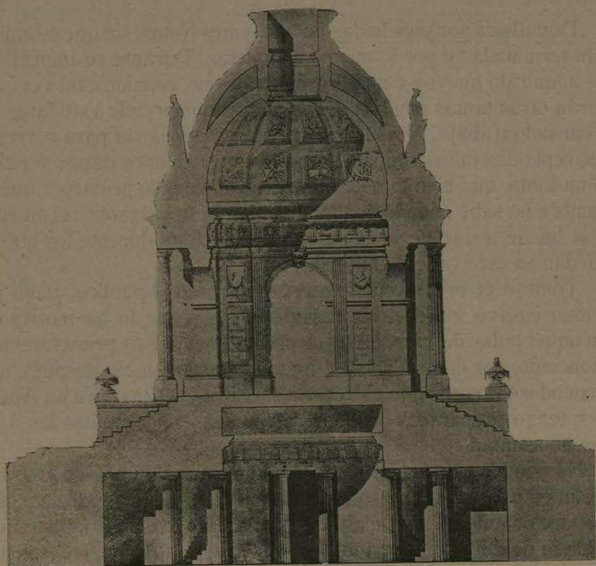
Corte del monumento central del Panteón Nacional, que actualmente se construye.
